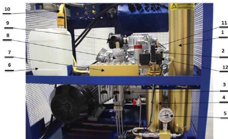
Рисунок 10- Блок осушки и очистки воздуха
