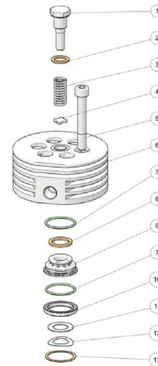
Рисунок 31 – Головка клапанов 3-й ступени
