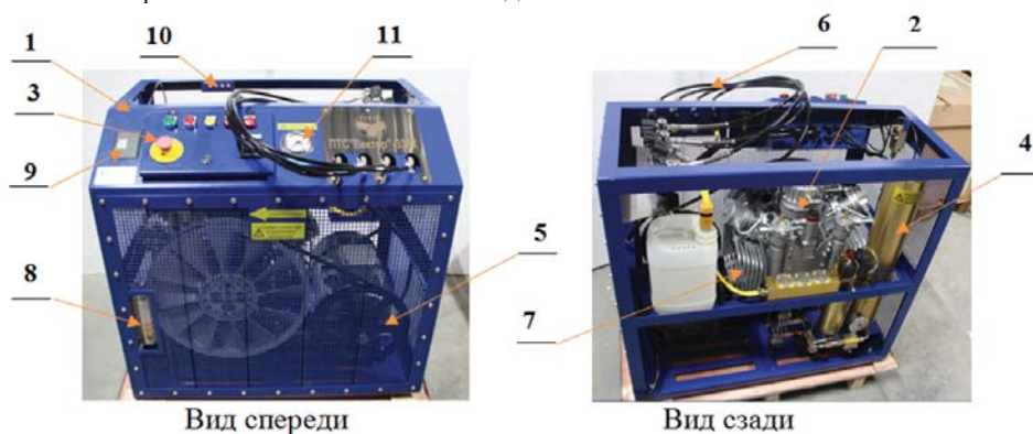
Рисунок 1- Основные узлы компрессора
