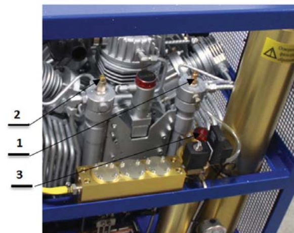
Рисунок 9- Предохранительные клапаны
