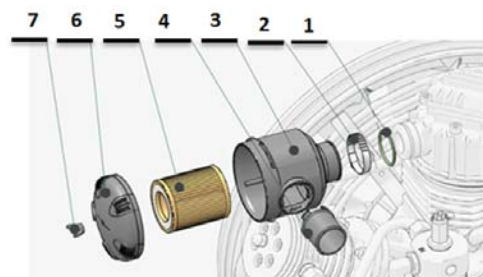
Рисунок 11- Входной воздушный фильтр грубой очистки
